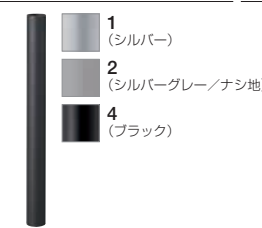
材質: スチール丸パイプ (60.5φ) 粉体塗装
